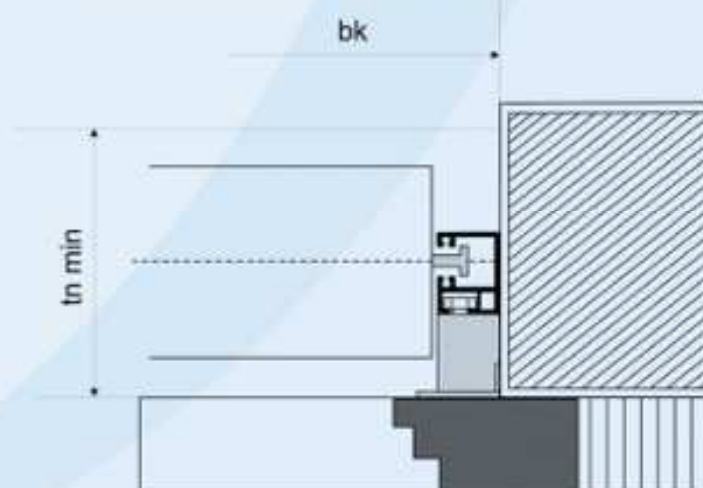
Presek solomatic-a sa vođicom
